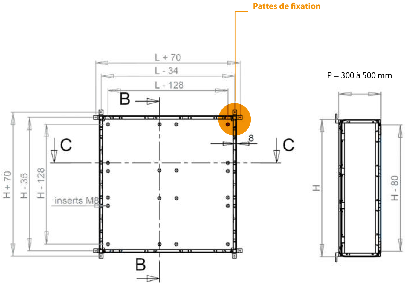
A-A (1:15)
