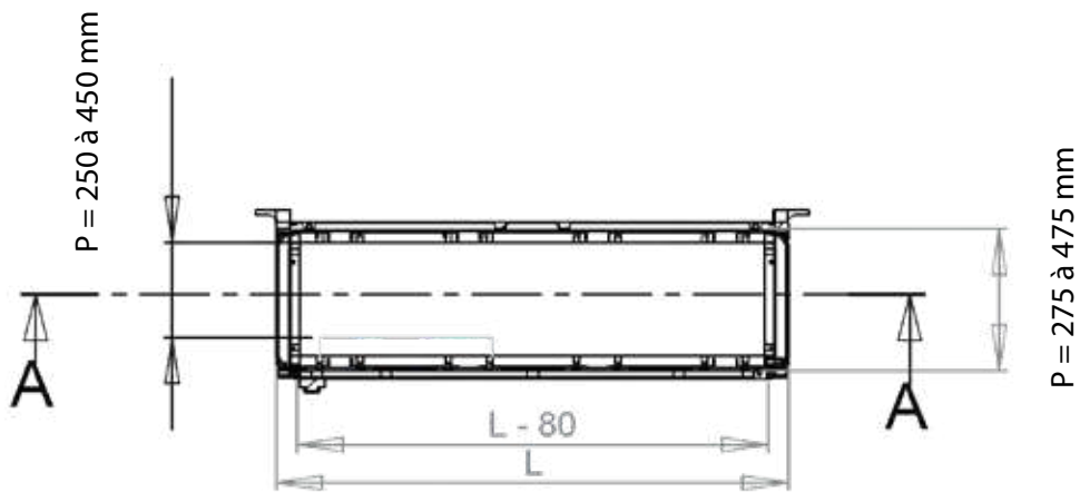
D-D (1:15)
